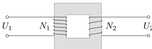
Рис. 2. Трансформатор
