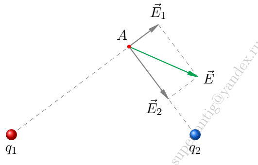
Рис. 1. Принцип суперпозиции для напряженностей
