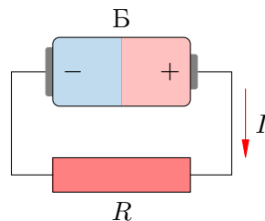
Рис. 1. Опыт с батарейкой и проводом
