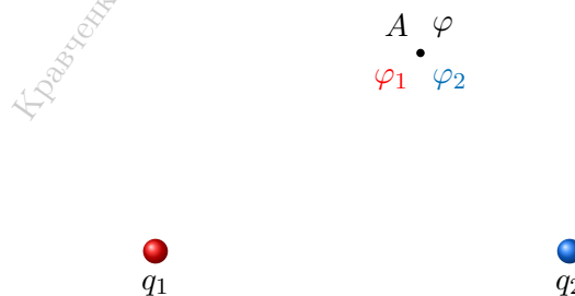
Рис. 2. Принцип суперпозиции для потенциалов
