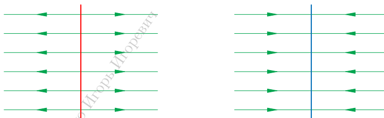
Рис. 2. Линии электрического поля заряженной пластины
