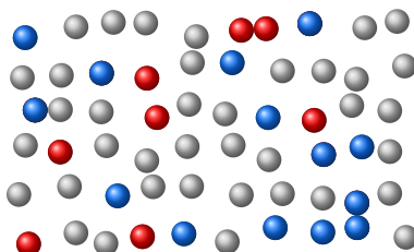
Рис. 2. Модель электролита (раствор)
