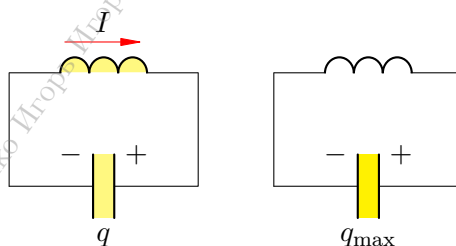
Рис. 2. Электромагнитные колебания в колебательном контуре
