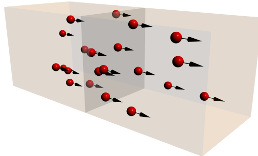
Рис. 1. Электрический ток
