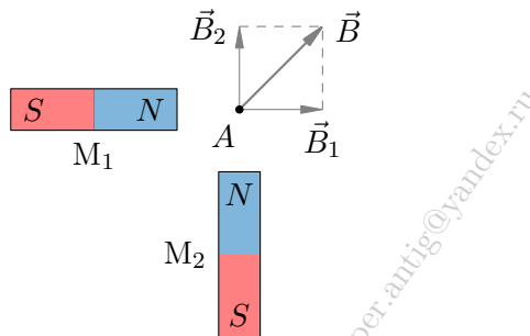
Рис. 1. Принцип суперпозиции магнитных полей
