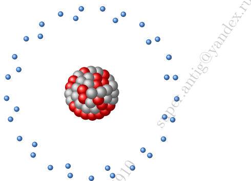
Рис. 1. Модель атома
