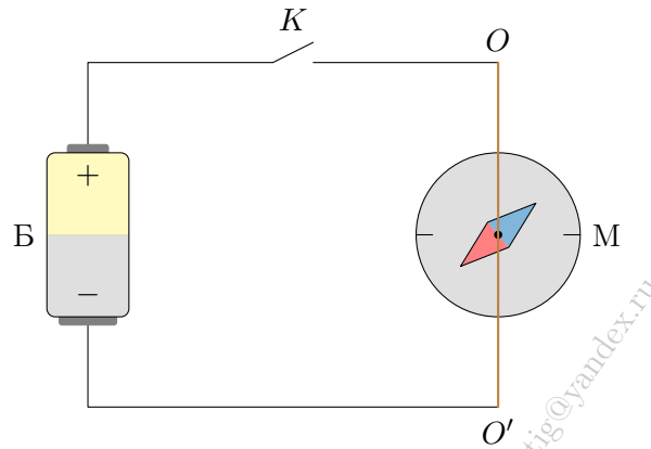
Рис. 1. Опыт Эрстеда: тока в цепи нет
