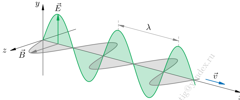
Рис. 1. Электромагнитная волна
