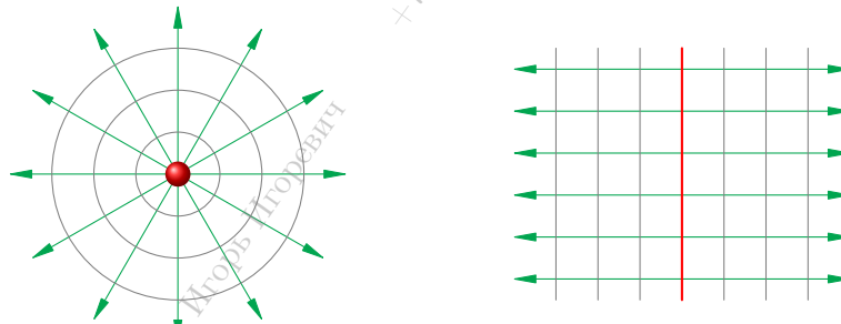
Рис. 2. Перпендикулярность эквипотенциальных поверхностей и линий поля
