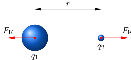
Рис. 1. Взаимодействие двух отрицательных зарядов
