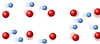
Рис. 2. Направленное движение электронов между ионами металла
