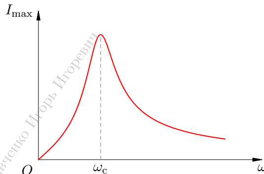
Рис. 2. Резонансная кривая
